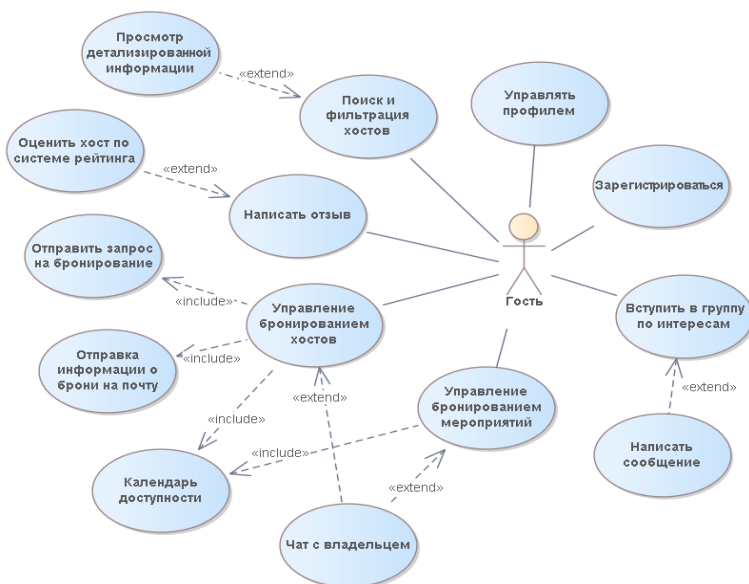
Рис. 2. Диаграмма вариантов использования
