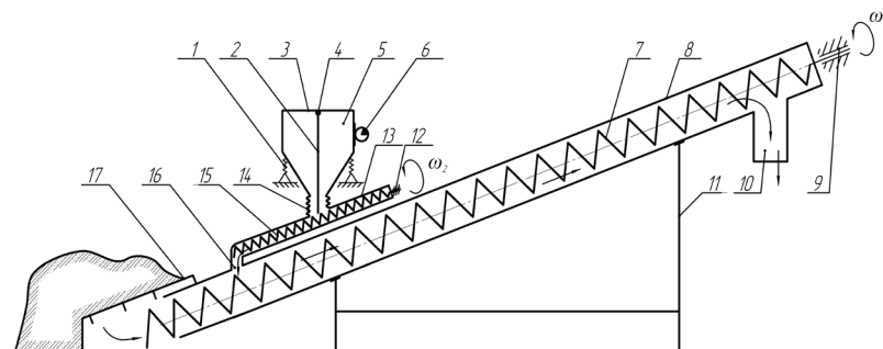
Рисунок 1 – Схема смесителя минеральных удобрений:
